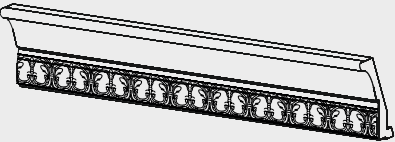
CORNICE MOULDING ВЕРХНИЙ КАРНИЗ 3000 x 132,5 x 30 (H 110)
